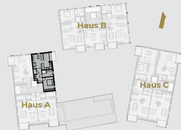
Zweites Obergeschoss - Etagenansicht
